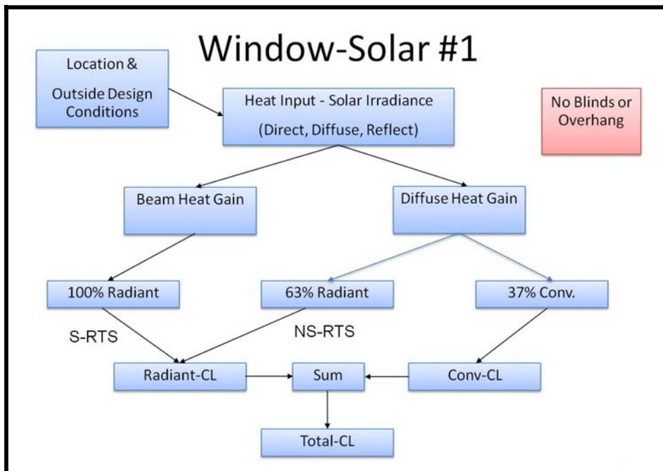
รูปที่ 9: Schematic Diagram แสดงขั้นตอนการคำนวณภาระความร้อนจากหน้าต่าง (กรณีที่มี 1)
